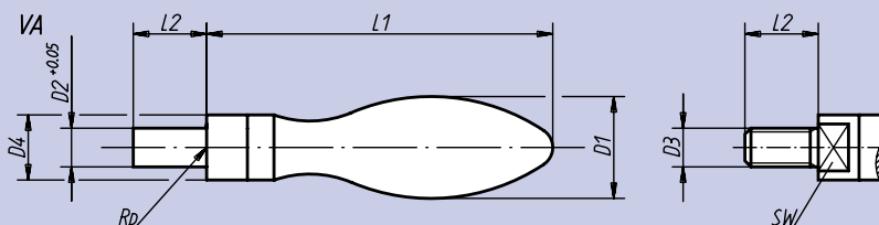
Forme D embout cylindrique
