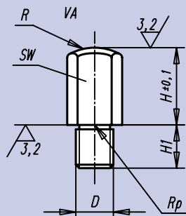
Forme C Surface bombée
