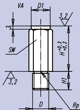
Forme C Surface bombée
