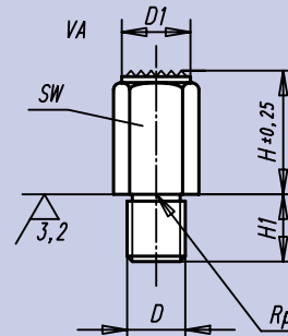
Forme D Surface à picots
