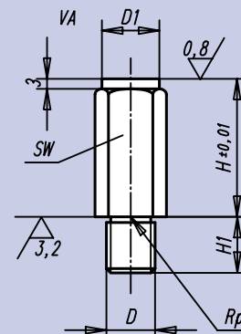
Forme D Surface à picots
